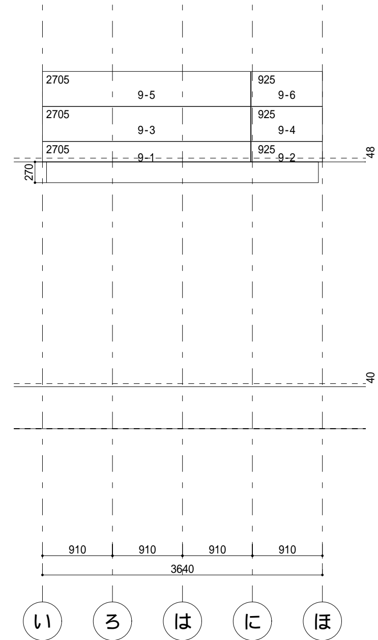
南面1通り割付図 S = 1 : 5 0
