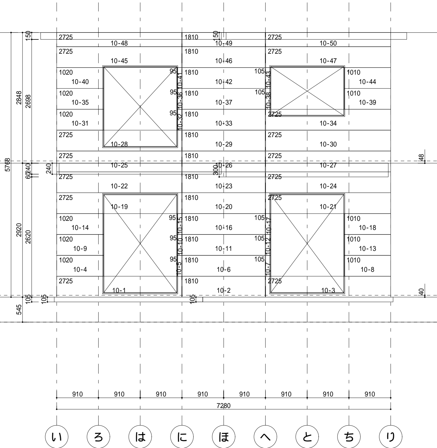
南面2通り割付図 S = 1 : 5 0
